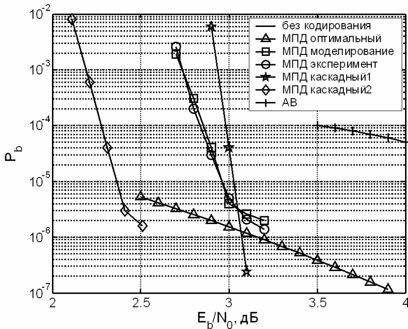
Рис. 1. Характеристики ПЛИС МПД сверточного кода канале с АБГШ
